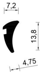
Brtva A - 0205
