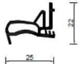
Brtva A- 0061
