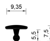
Brtva A - 0204
