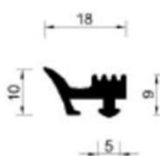
Brtva B-1025
