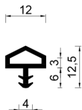
Brtva D-0002
