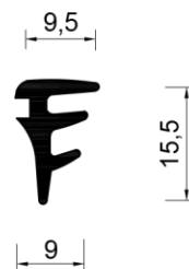
Brtva A - 0206
