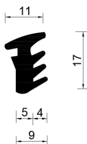
Brtva A - 0203
