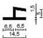
Brtva A-0108
