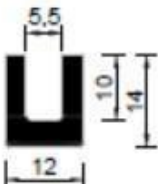
Brtva A-0094
