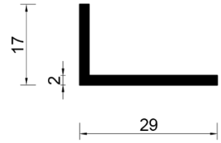
Brtva A- 0107
