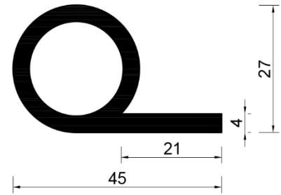
Brtva P - 0002
