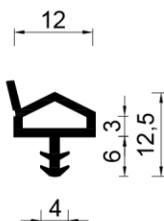
Brtva D-0003
