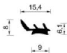
Brtva A-0004
