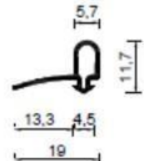
Brtva A- 0168
